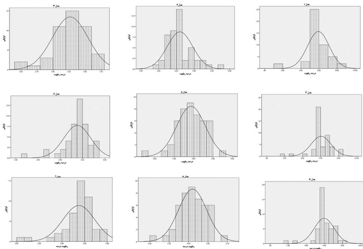
شکل ۴: هیستوگرام و منحنی برازش داده‌شده‌ی خطا در هر مدل
