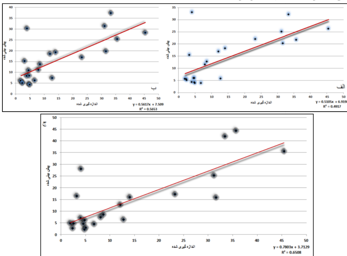
شکل ۹: نمودار پراکندگی مقادیر برآوردی و مشاهده‌ای سه روش الف IDW، ب: کریجینگ، ج: Completely Regularized spline
