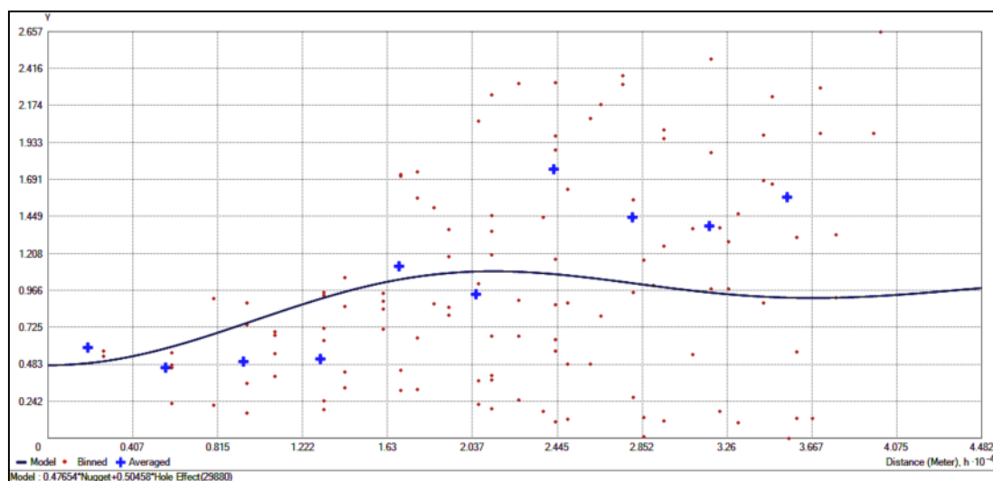
شکل ۷: منحنی نیم تغییرنمای محاسبه شده‌ی روش کریجینگ با مدل نظری برازش داده شده به آن
