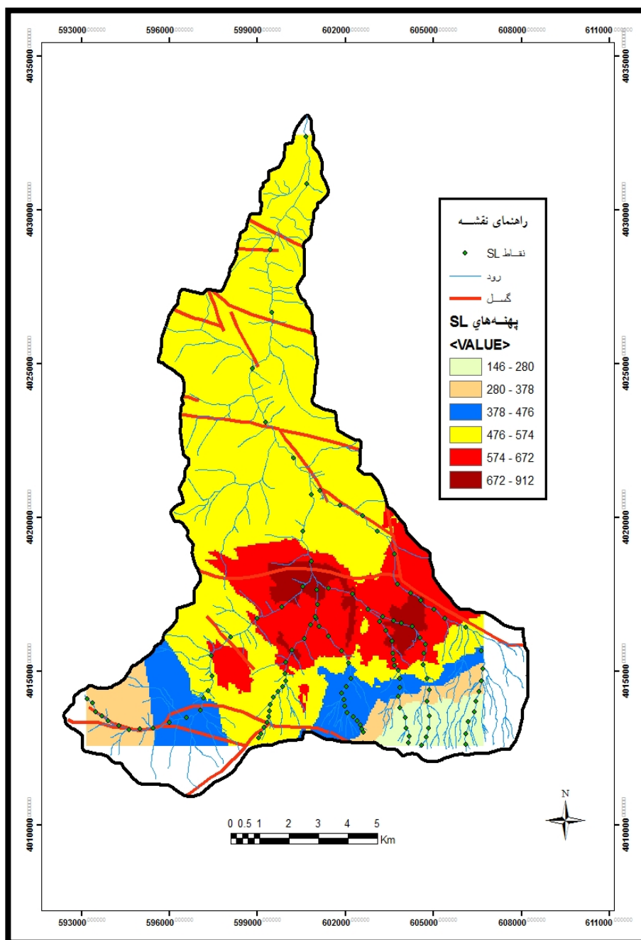
شکل ۷. نقشه‌ی گرادیان طولی (SL) شبکه‌های زهکشی حوضه‌ی آبریز واز
