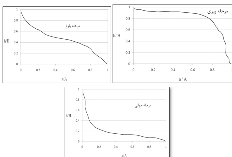
شکل ۴: منحنی‌های هیپسومتری نظری چرخه فرسایش کلا و همکاران، ۲۰۰۲
